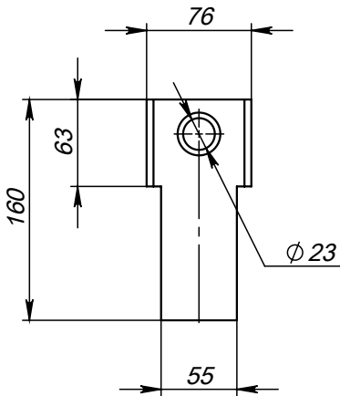
Поз.5 (Пластина)
